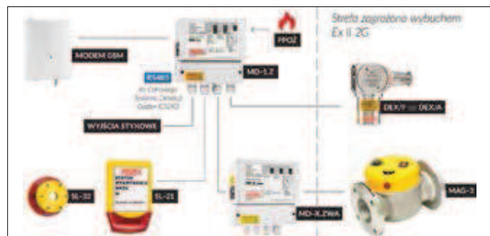
Modularny System Detekcji Gazu GAZEX
